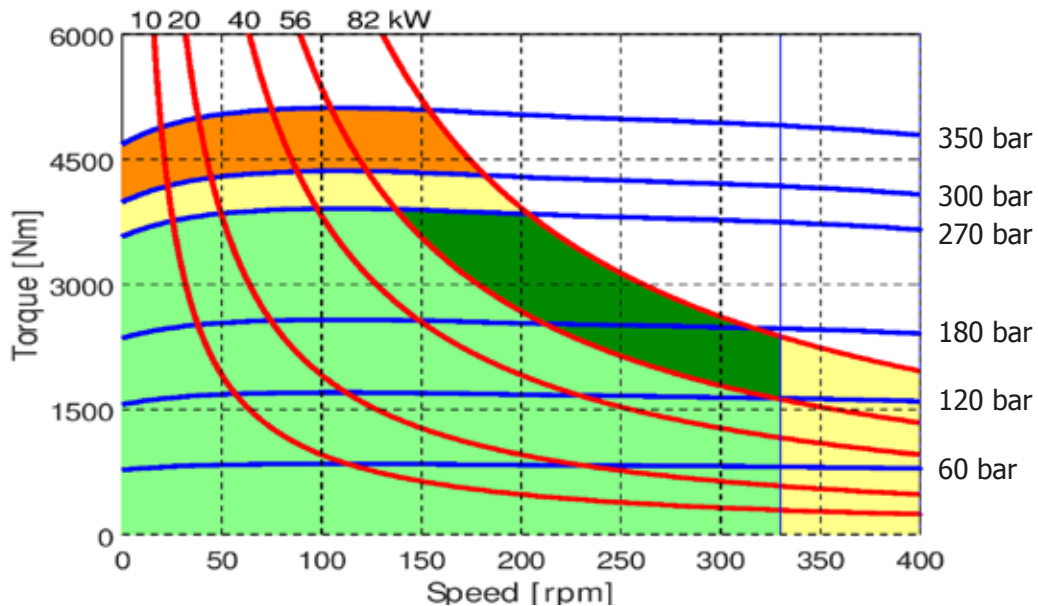
R8M 1100 H4
