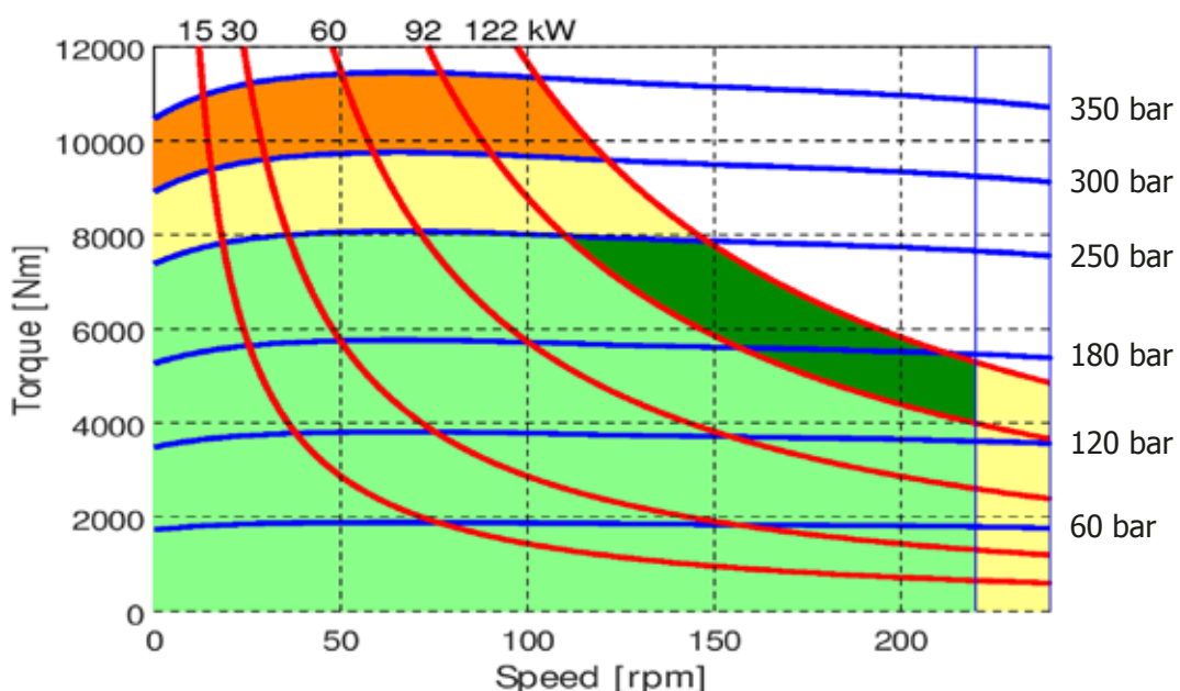
R8M 2200 H5
