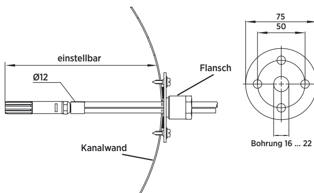
Links: Kanalinstallationssatz Rechts: Montageflansch. Aluminium oder Edelstahl.
