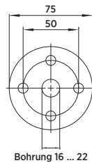
Sonde HMP375 und Montageflansch aus Edelstahl. Abmessungen in mm.
